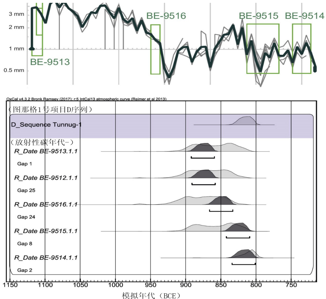
图5: 样品的测量段和同步平均树木年轮年代学曲线, 包括用于放射性碳测年的取样环段(上)。树轮层的放射性碳年代分布(下)。
