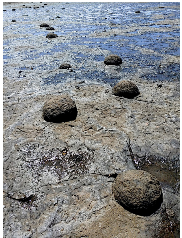
图5: 新南威尔士州南海岸阿勒达拉(Ulladulla)的石弹地貌(Robert Bednarik jun摄)。
